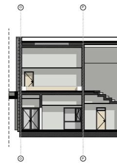
Schnitt Sporthalle
