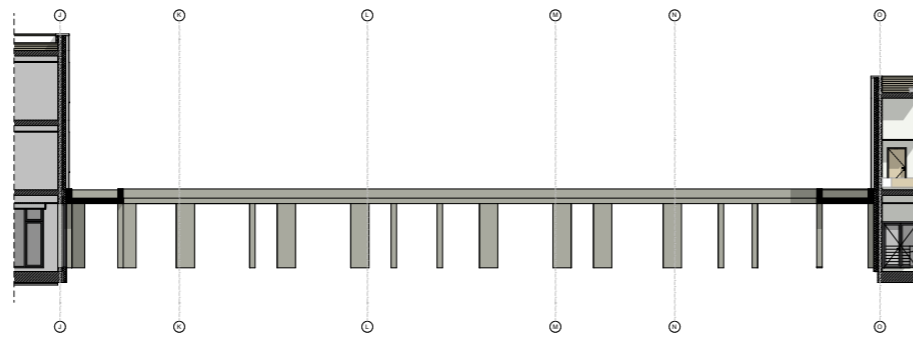
Ansicht Süd Laubengang
