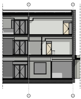
Schnitt Schule
