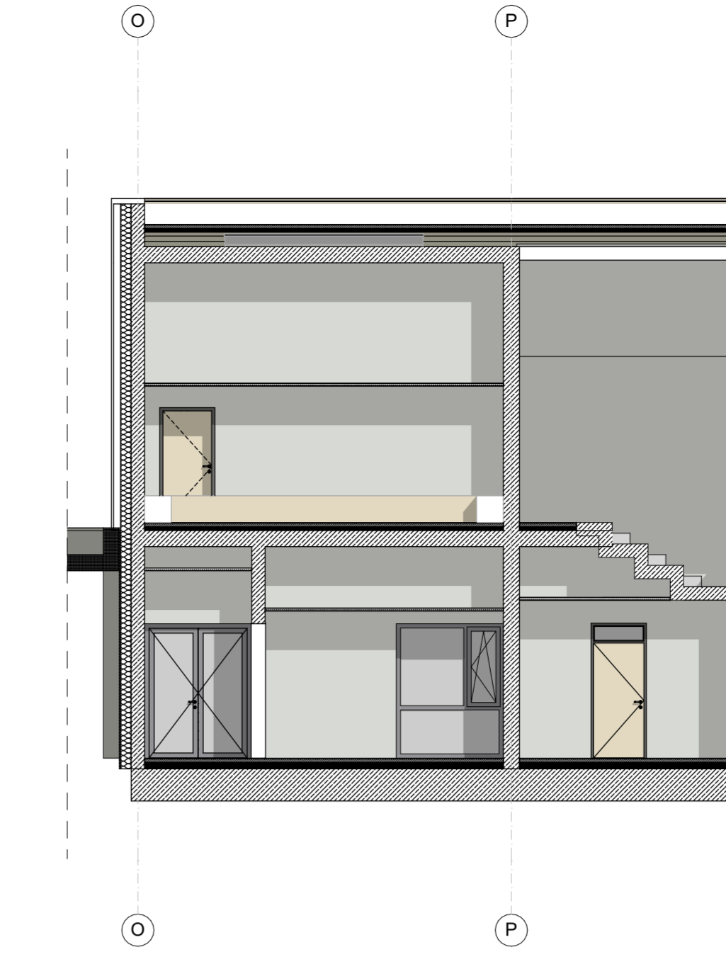
Schnitt Sporthalle
