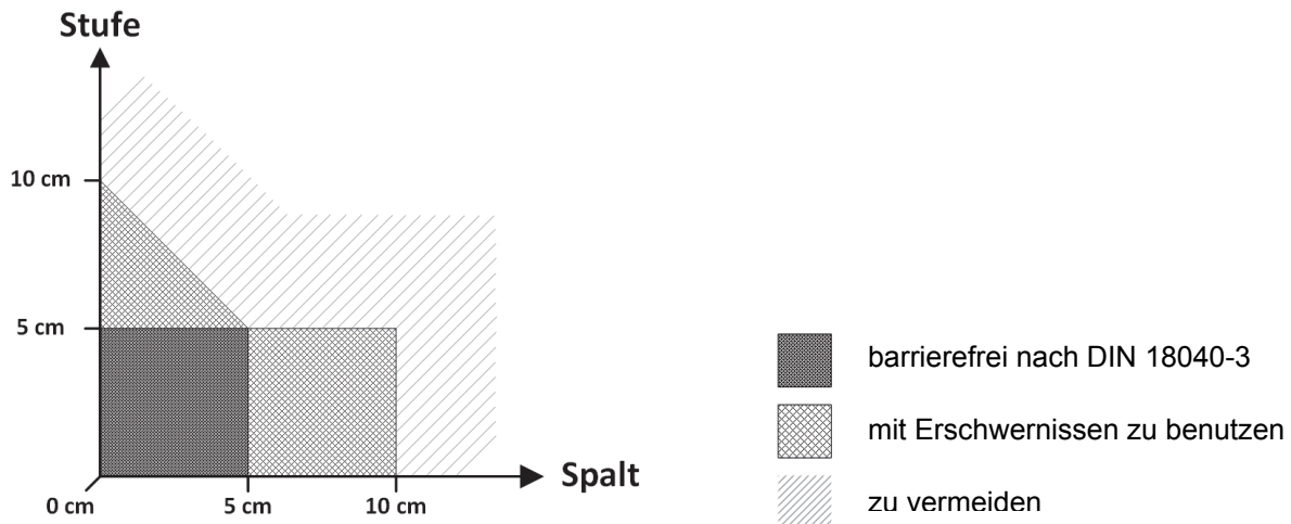
Abbildung 7: Empfohlene Reststufenhöhe und Spaltbreite (verändert nach: Bundesministerium für Verkehr 1997, S.24)
