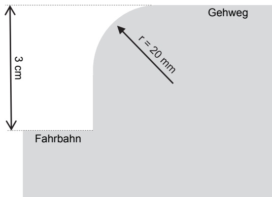
Abbildung 6: Ausrundung einer 3 cm Bordkante mit r = 20 mm (verändert nach: Boenke et al. 2014, S.82)
