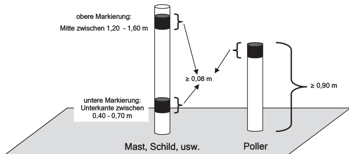
Abbildung 1: Visuelle Kennzeichnung von Hindernissen (verändert nach Forschungsgesellschaft für Straßen- und Verkehrswesen e. V. - Arbeitsgruppe Straßenentwurf 2011, S.30)
